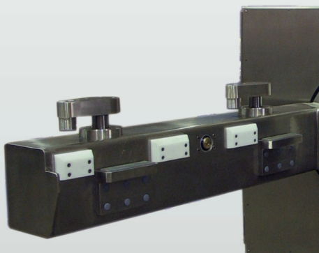
Blocage automatisé par quatres vérins de blocage pivotants et deux vérins de centrage latéraux
